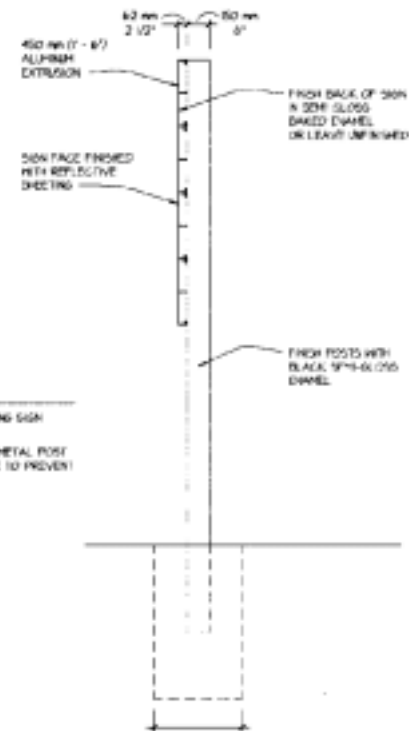
SECTION SCALE: 1/4"=1'-0"
